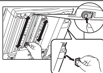
Podávacie valček na papier
